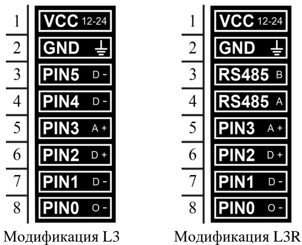
Рисунок 1 – Распиновка разъёма
