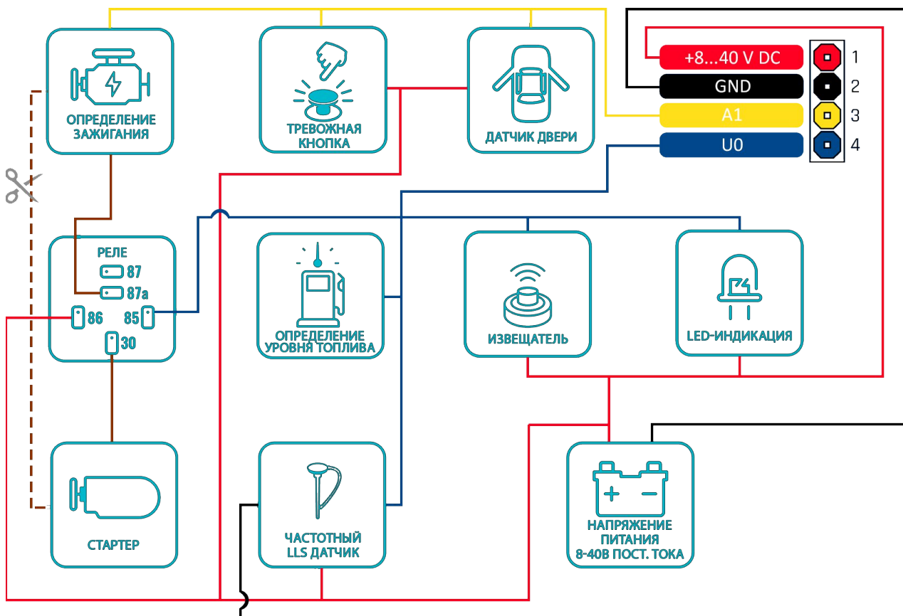
Рисунок 3. Базовая схема подключения
