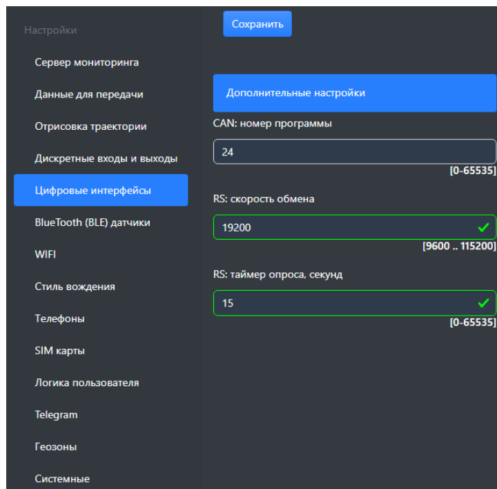
Рисунок 3 – дополнительные настройки цифровых интерфейсов
