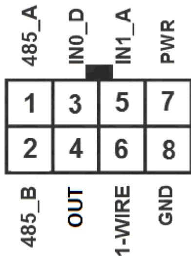
Рис 2. Общий вид основного разъема.
